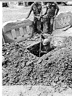
Construcción de pozos de lanzamiento
