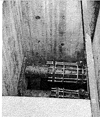
Terminación de la construcción de canal de lavado y cámaras de las válvulas de lavado.
