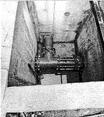
Terminación de la construcción de canal de lavado y cámaras de las válvulas de lavado.
