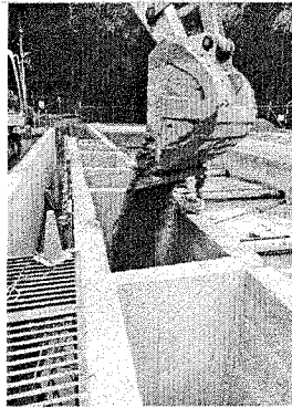
Relleno entre cámaras del sistema de lavado
