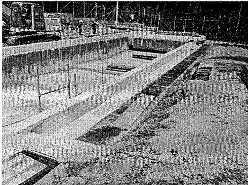
Fundición viga – Realce de muros
