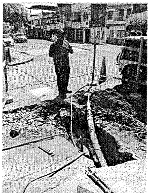
Traslado de acometidas domiciliarias
