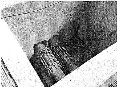
Instalación de niples pasamuros y válvulas
